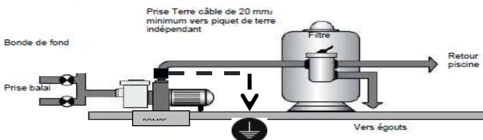
Montage d'une prise terre
